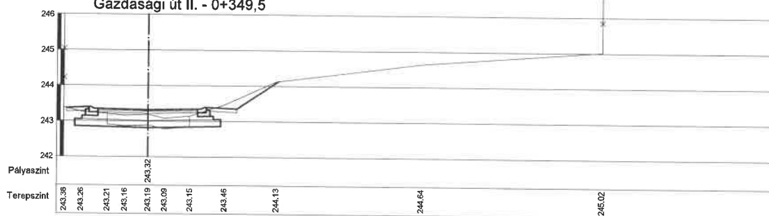
Gazdasági út II. - 0+349,5
