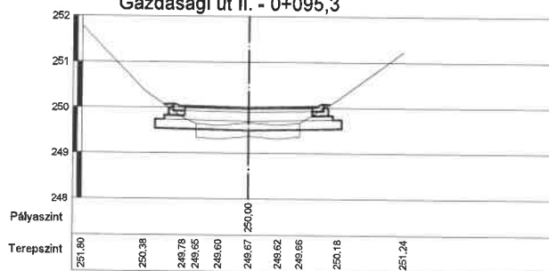
Gazdasági út II. - 0+095,3
